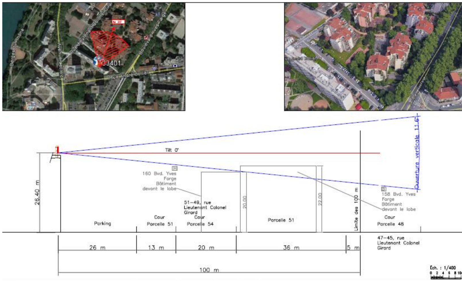
VUE EN COUPE DE L'AZIMUT 20°
