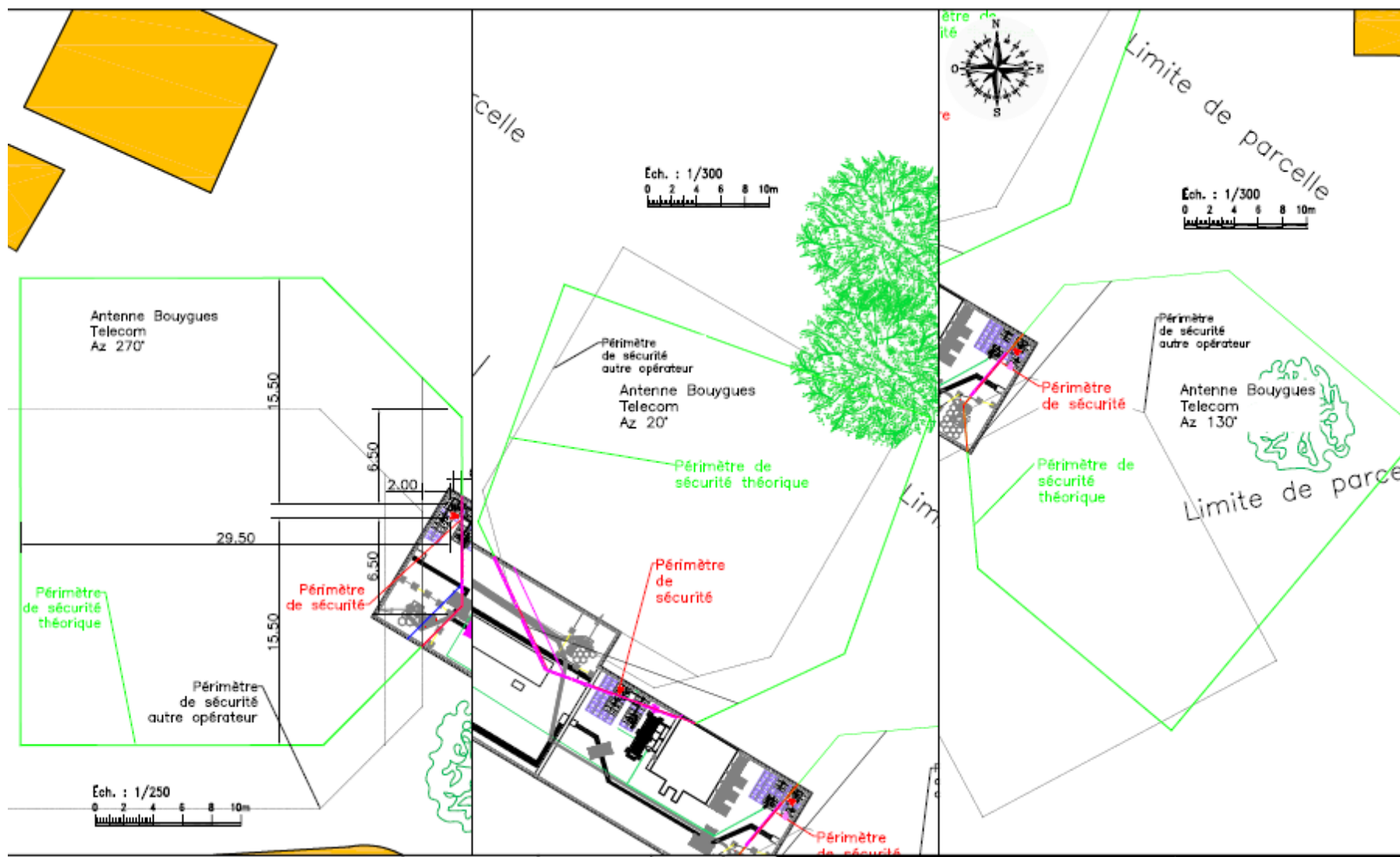
PERIMETRE DE SECURITE AUTOUR DE L'ANTENNE
