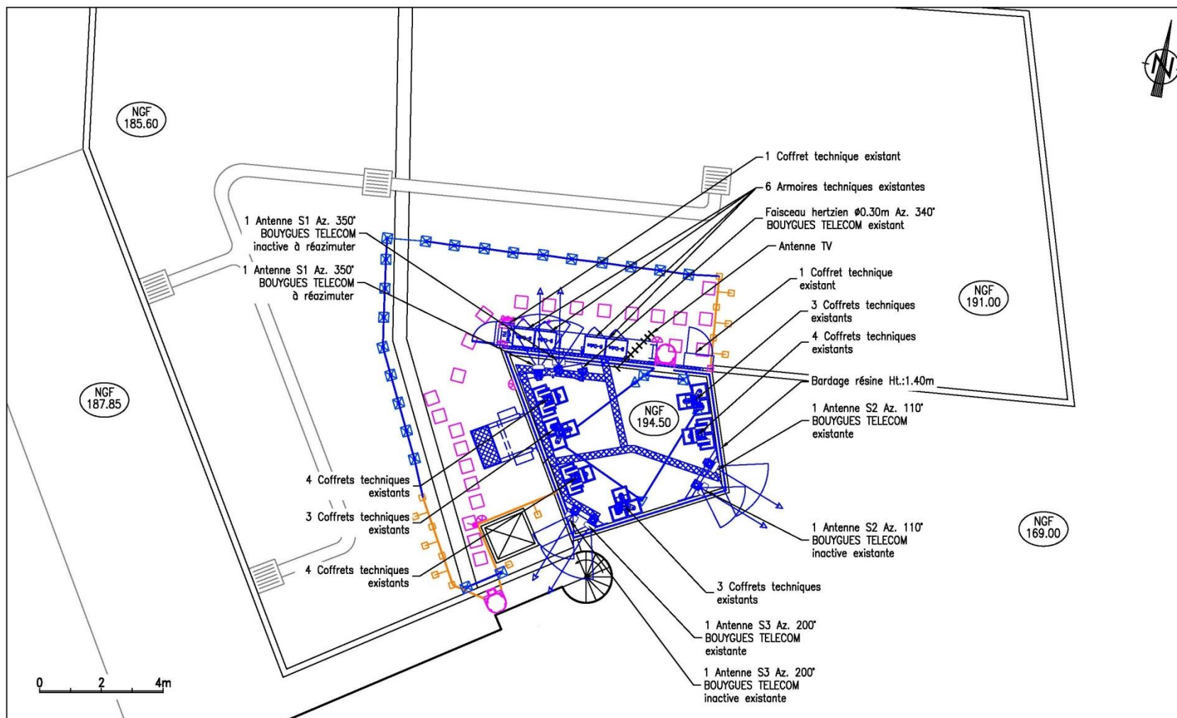
PLAN DE MASSE ETAT EXISTANT
