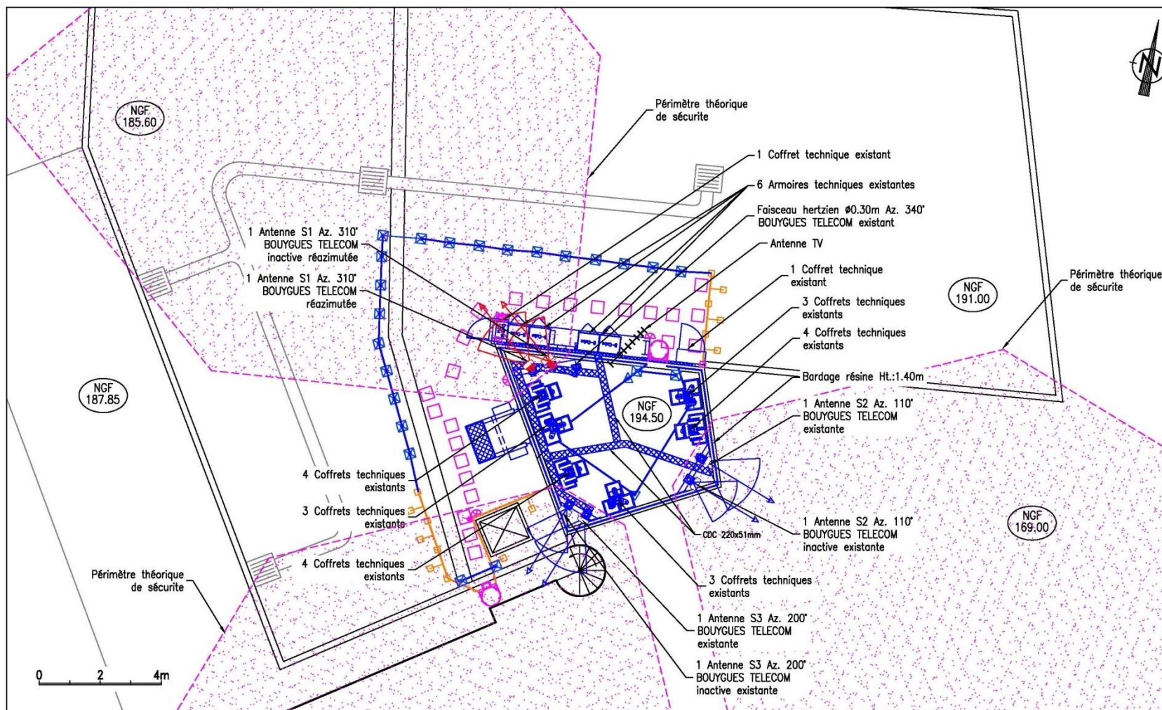
PERIMETRE DE SECURITE AUTOUR DES ANTENNES
