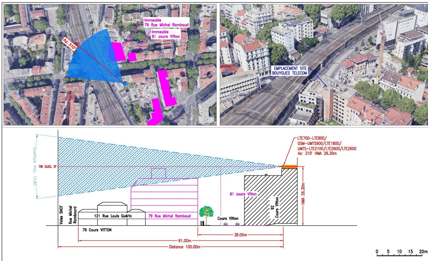
COUPE SUR L'AZIMUT 310°
