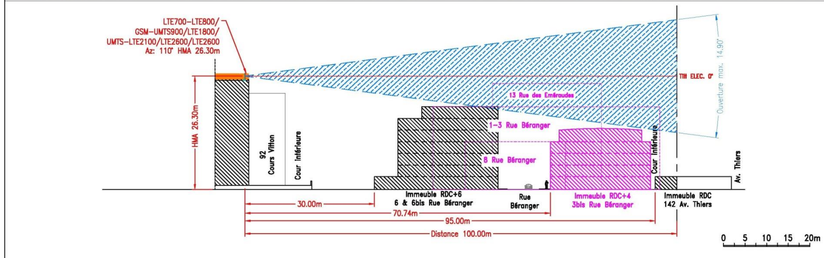
COUPE SUR L'AZIMUT 110°
