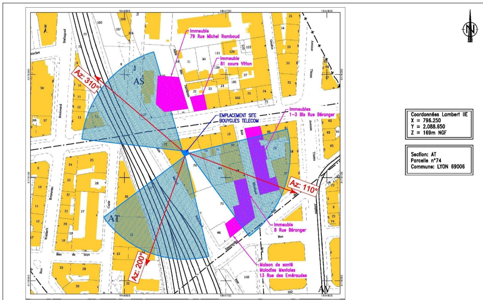
PLAN DE MASSE AVEC AZIMUT ET LOCALISATION DES ETABLISSEMENTS PARTICULIERS
