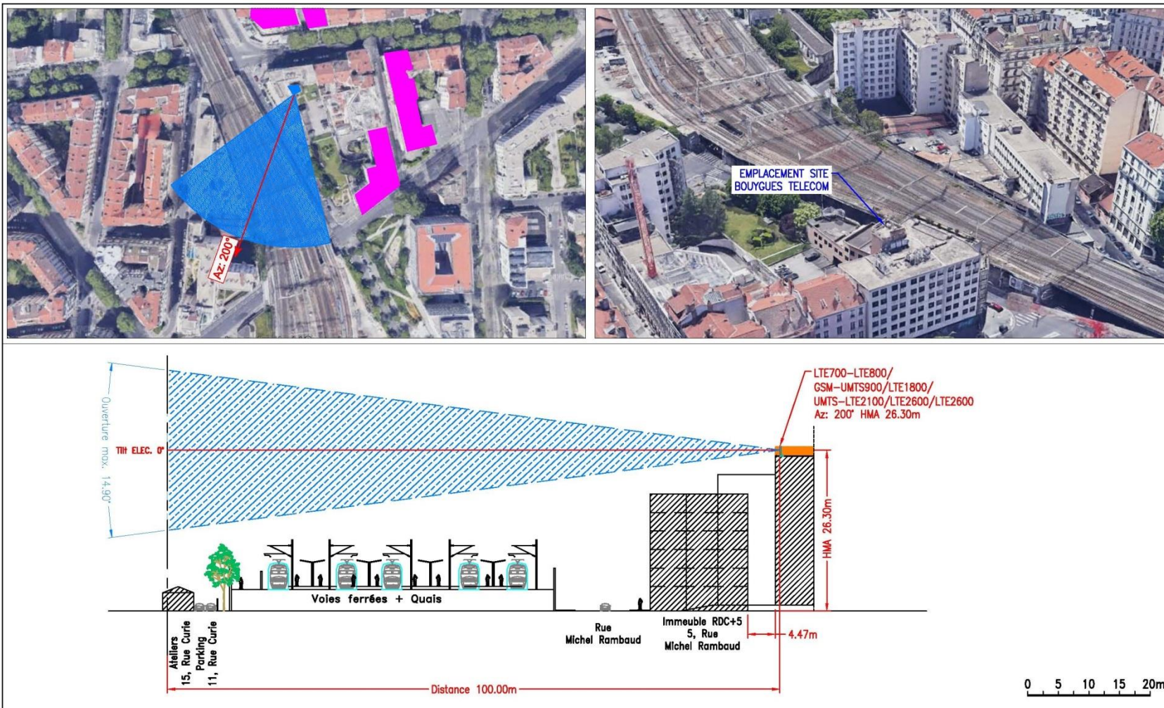
COUPE SUR L'AZIMUT 200°
