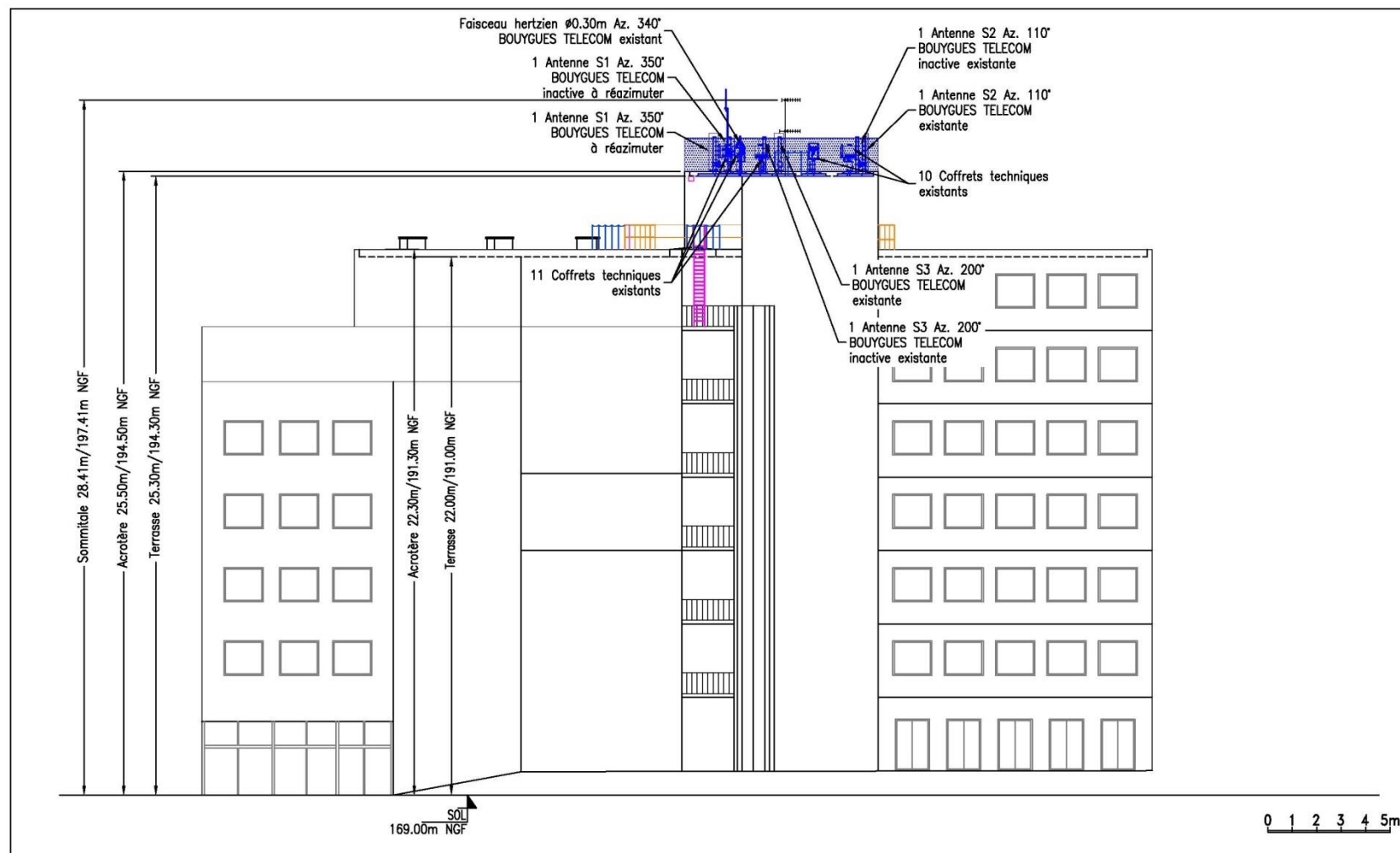
VUE EN ELEVATION ETAT EXISTANT
