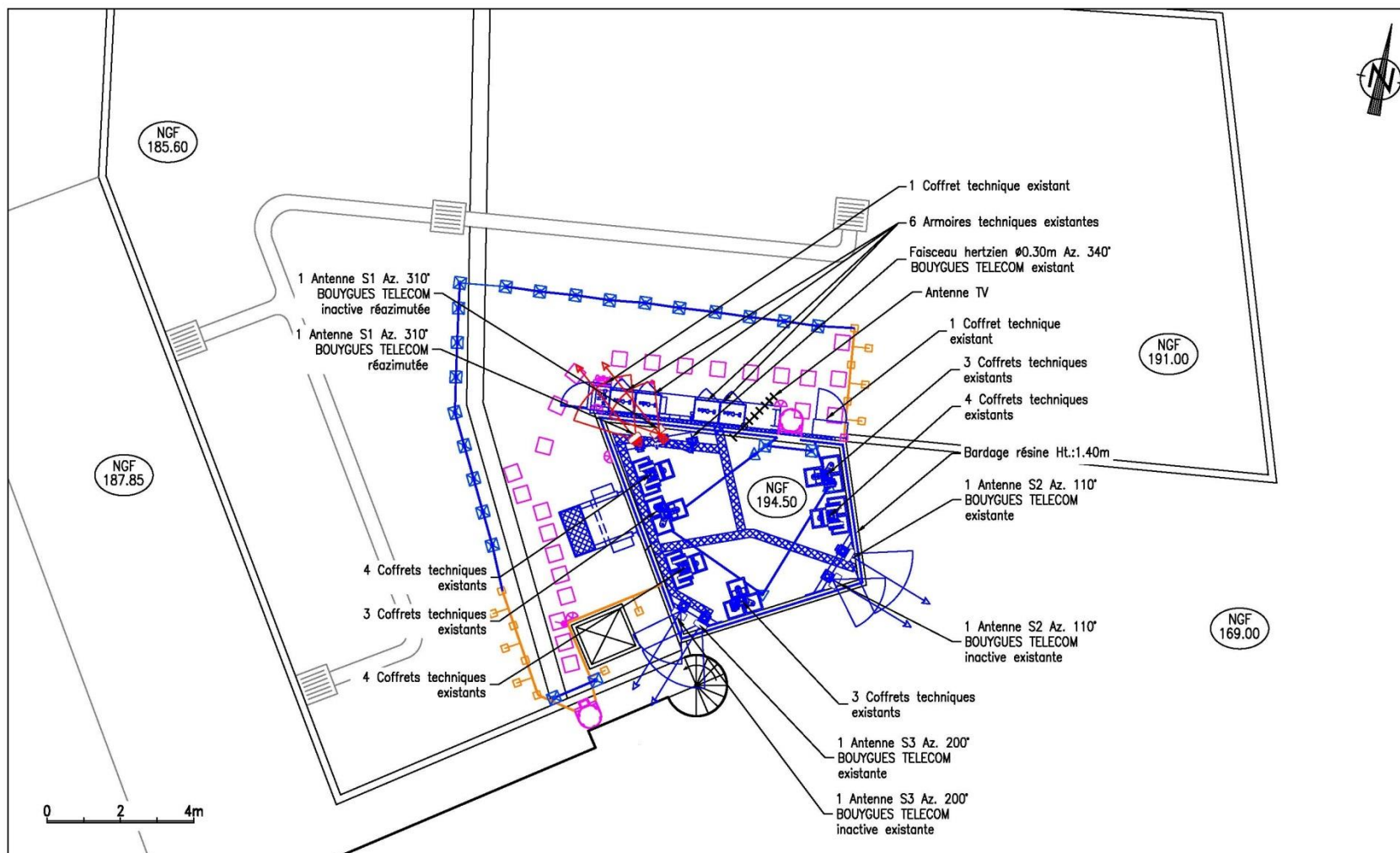
PLAN DE MASSE ETAT PROJETE
