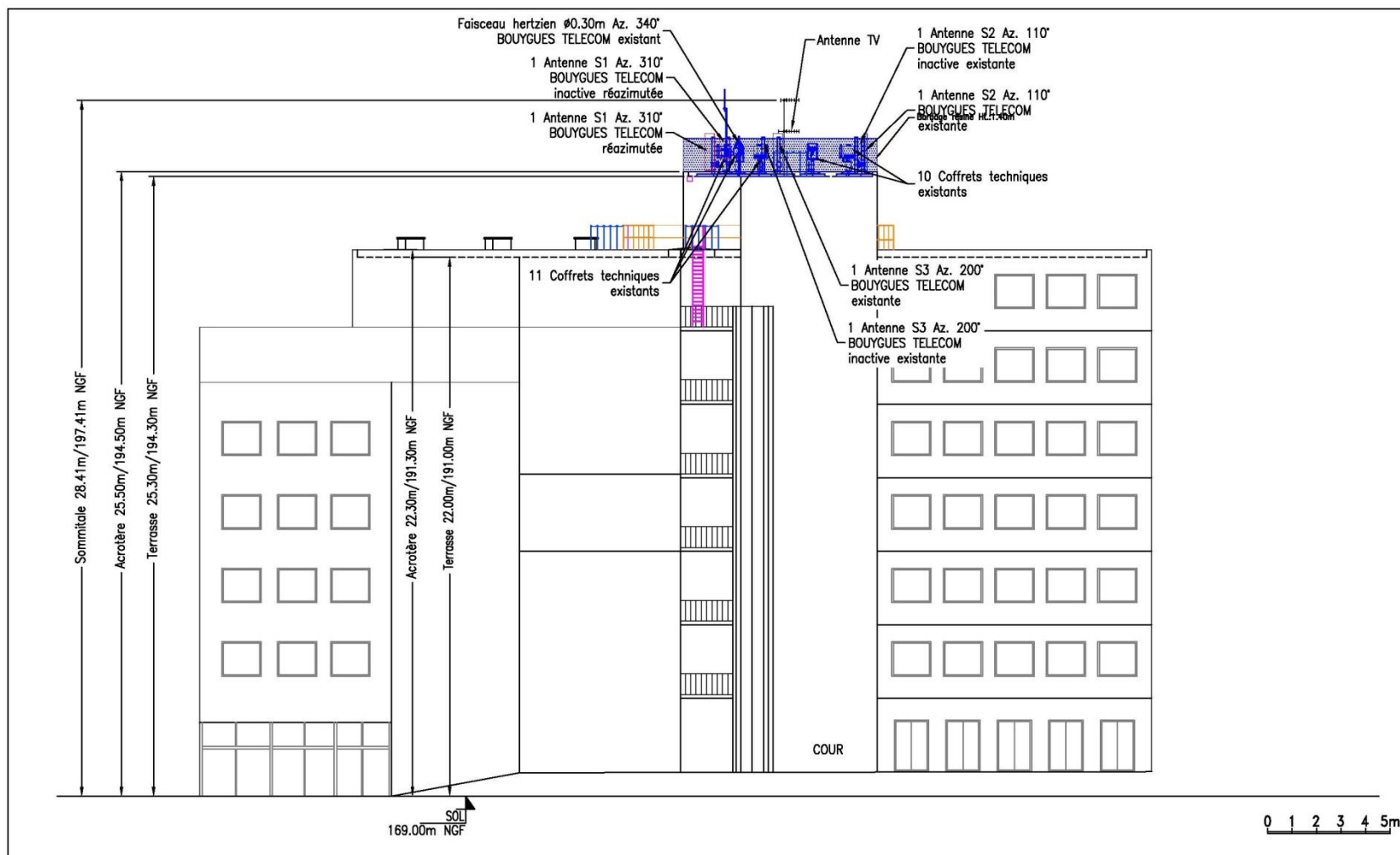
VUE EN ELEVATION ETAT PROJETE
