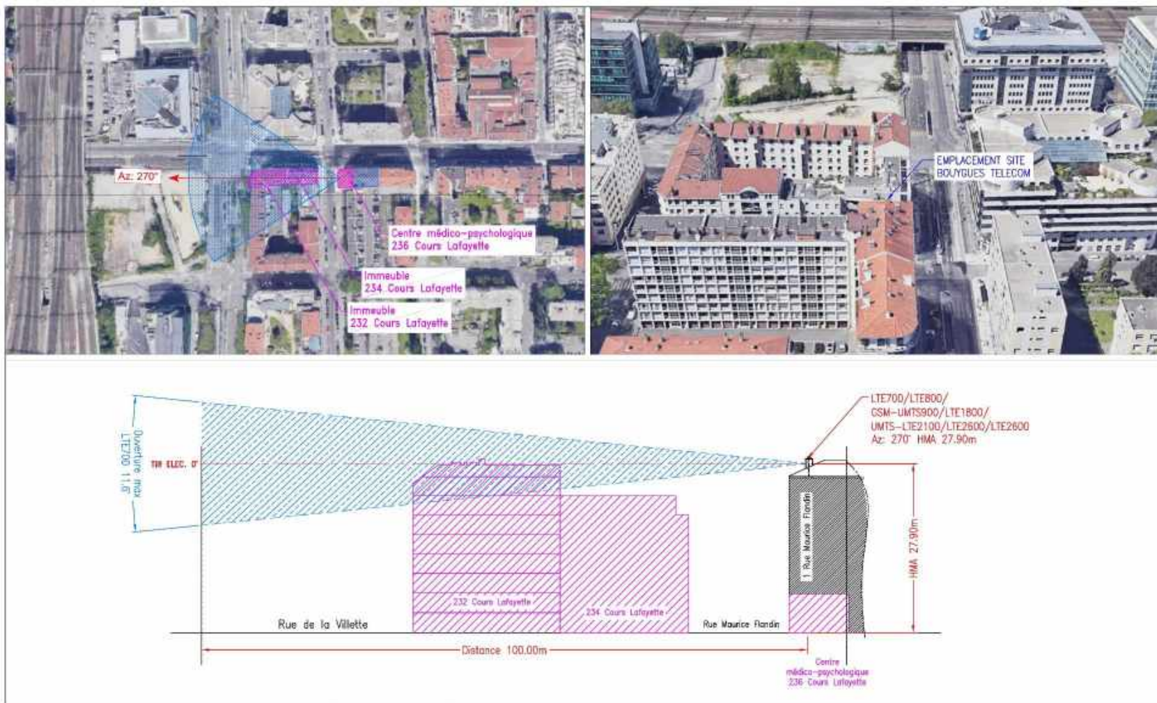
COUPE SUR L'AZIMUT 270°
