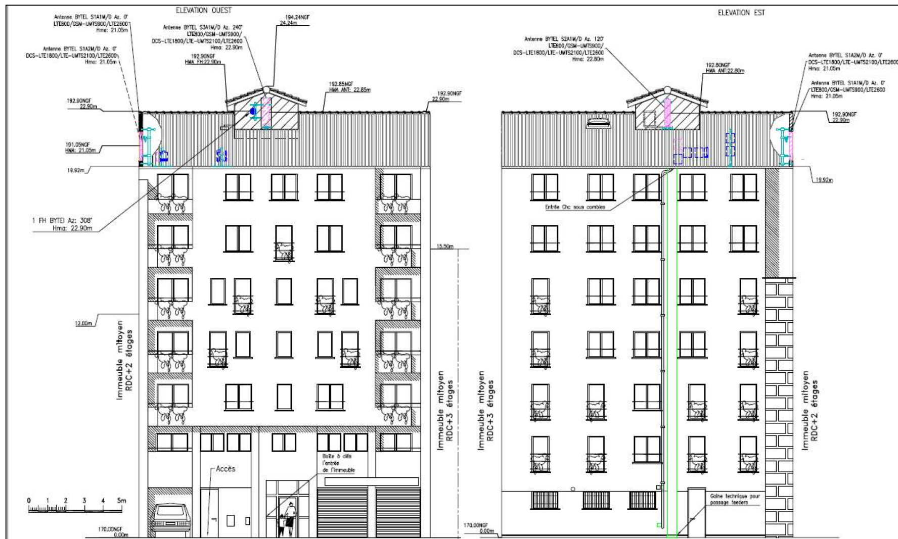
VUE EN ELEVATION ETAT EXISTANT
