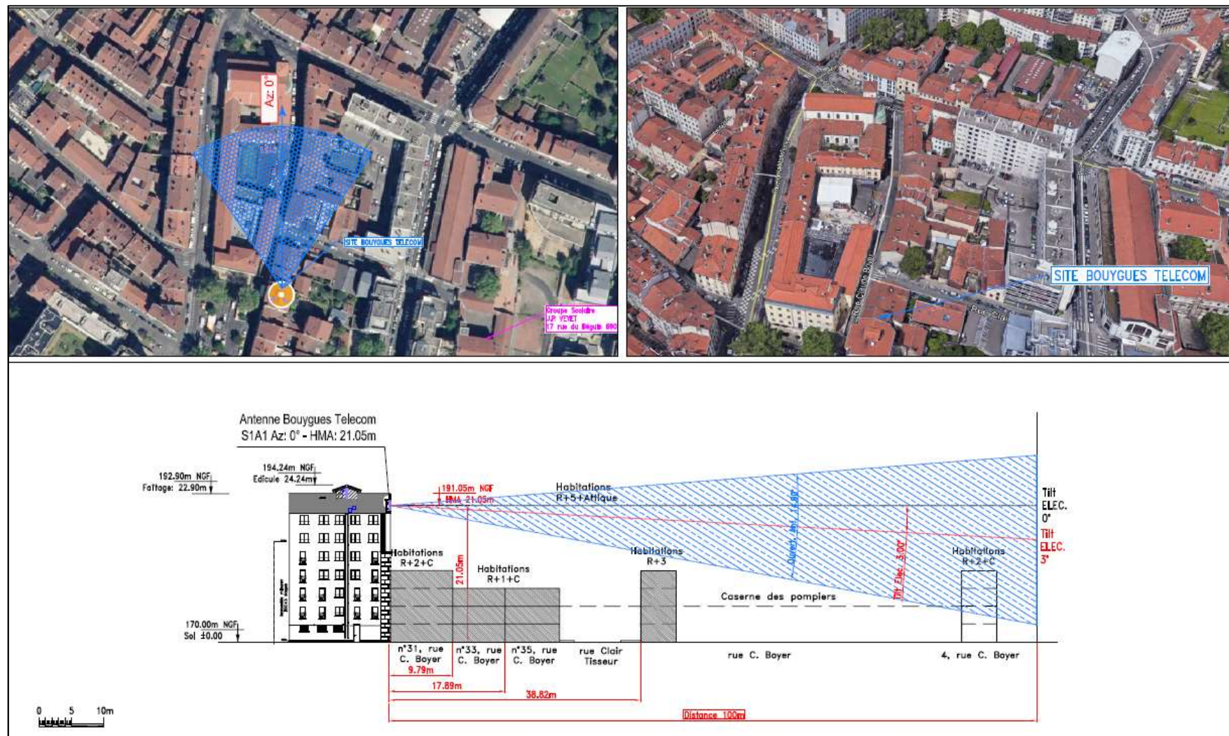
COUPE SUR L'AZIMUT 0°
