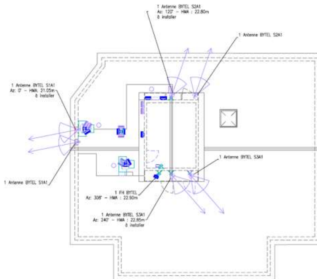
PLAN DE MASSE ETAT PROJETE
