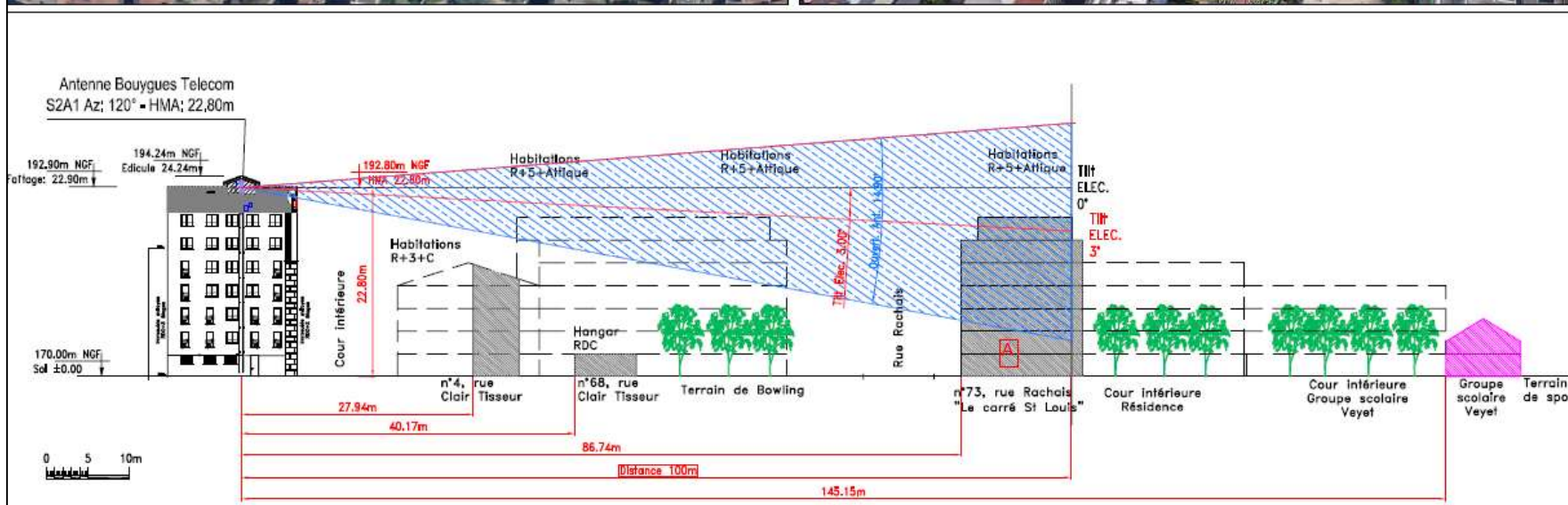
COUPE SUR L'AZIMUT 120°
