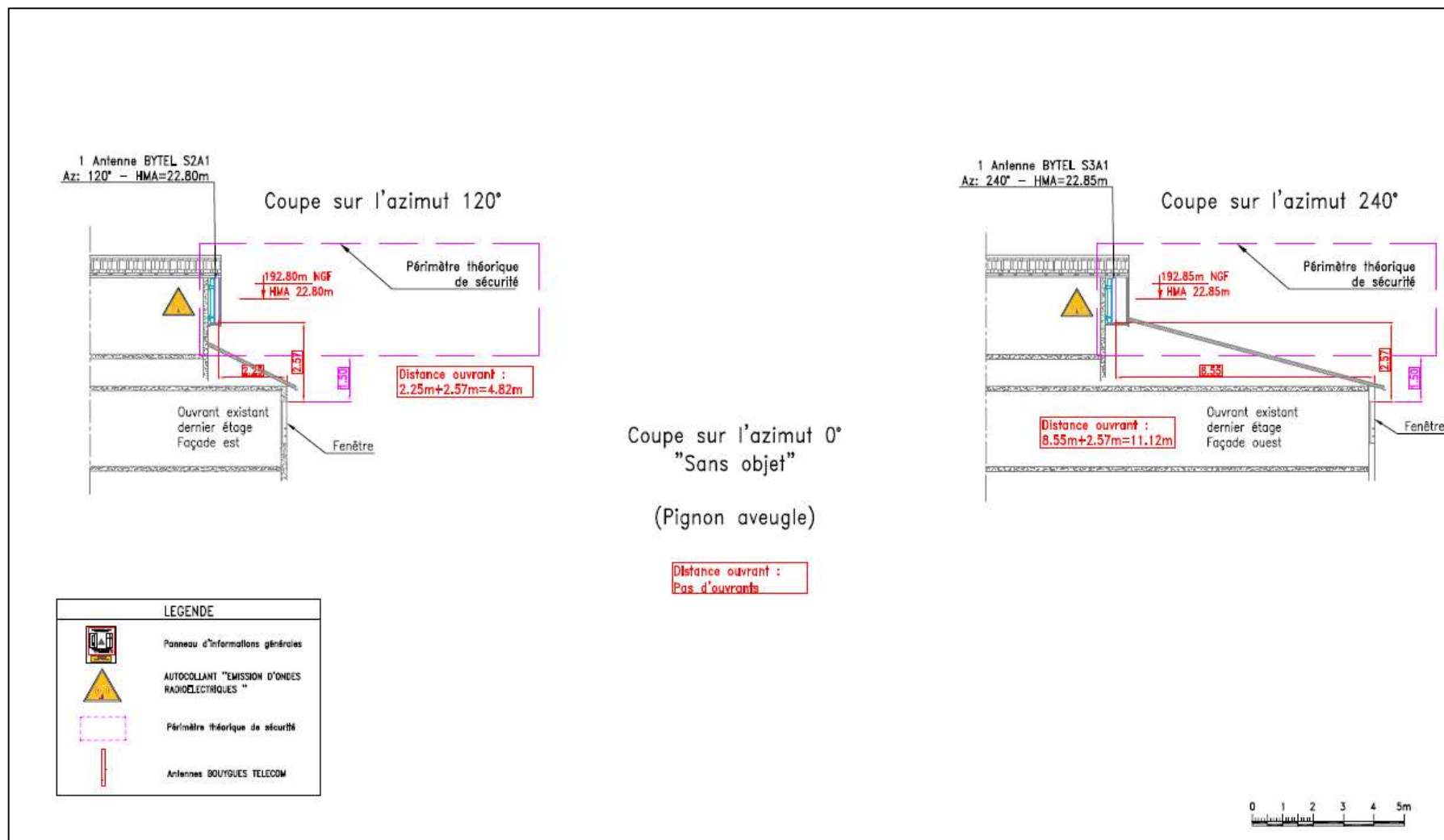
DISTANCE AUX OUVRANTS POUR CHAQUE AZIMUT
