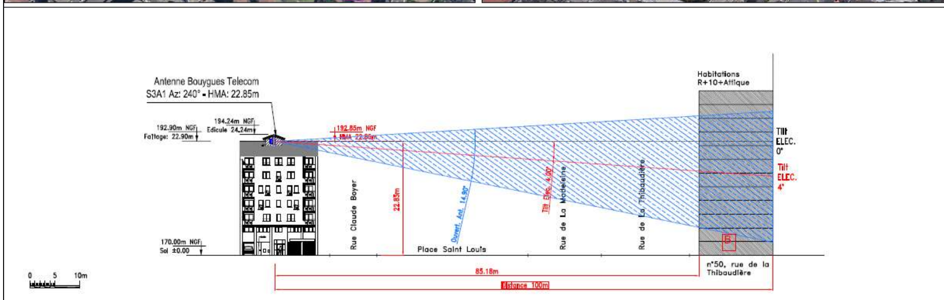
COUPE SUR L'AZIMUT 240°
