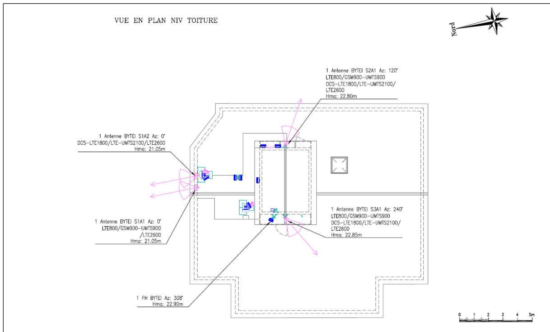
PLAN DE MASSE ETAT EXISTANT
