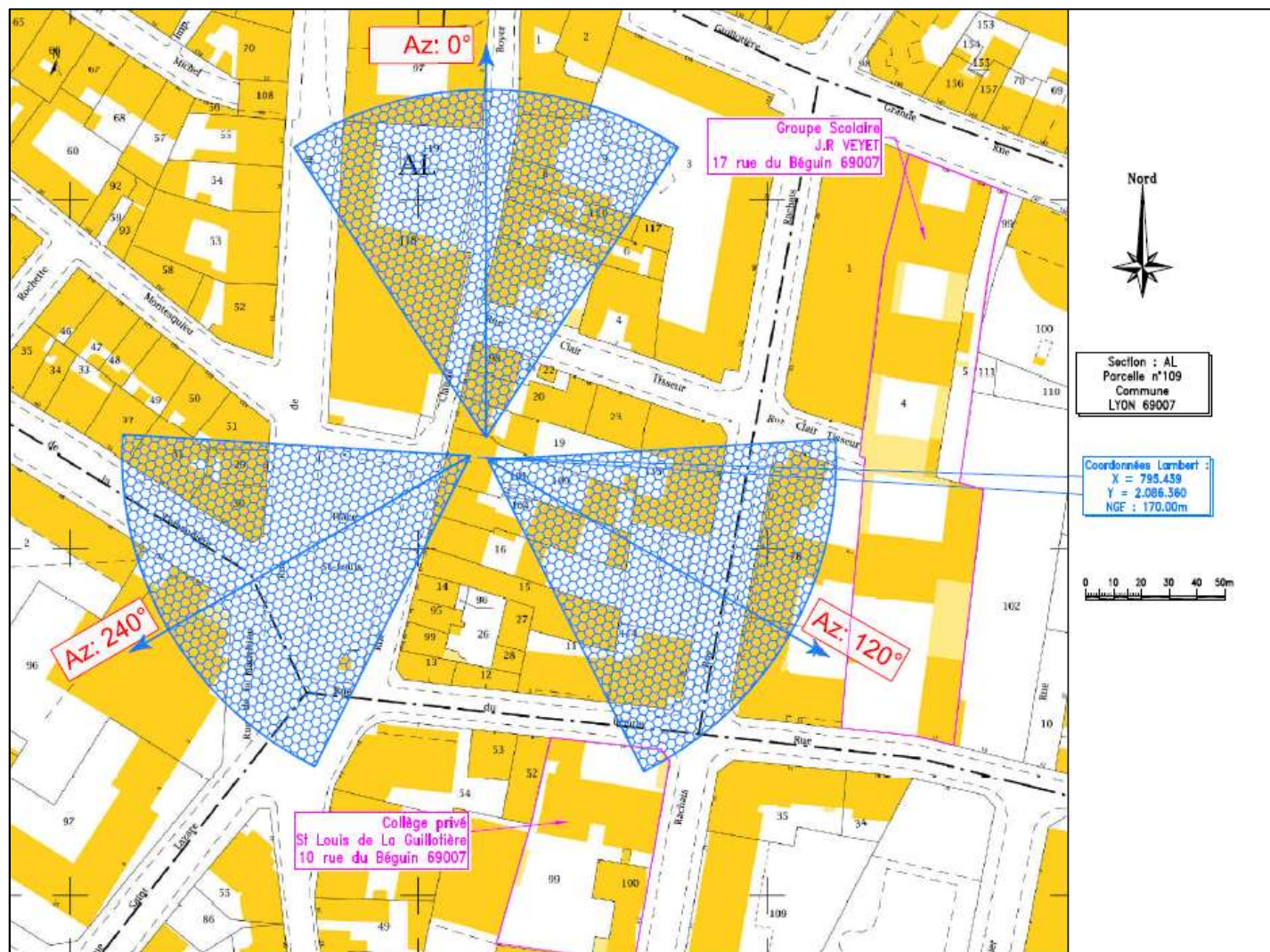
PLAN DE MASSE AVEC AZIMUTS ET LOCALISATION DES ETABLISSEMENTS PARTICULIERS
