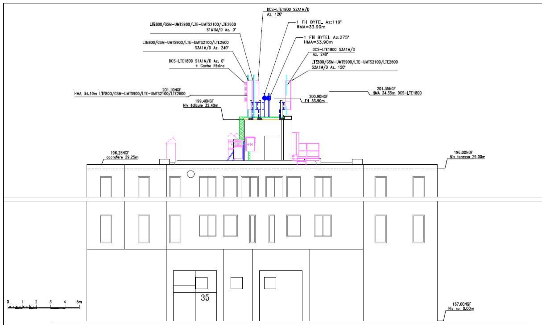
VUE EN ELEVATION ETAT EXISTANT
