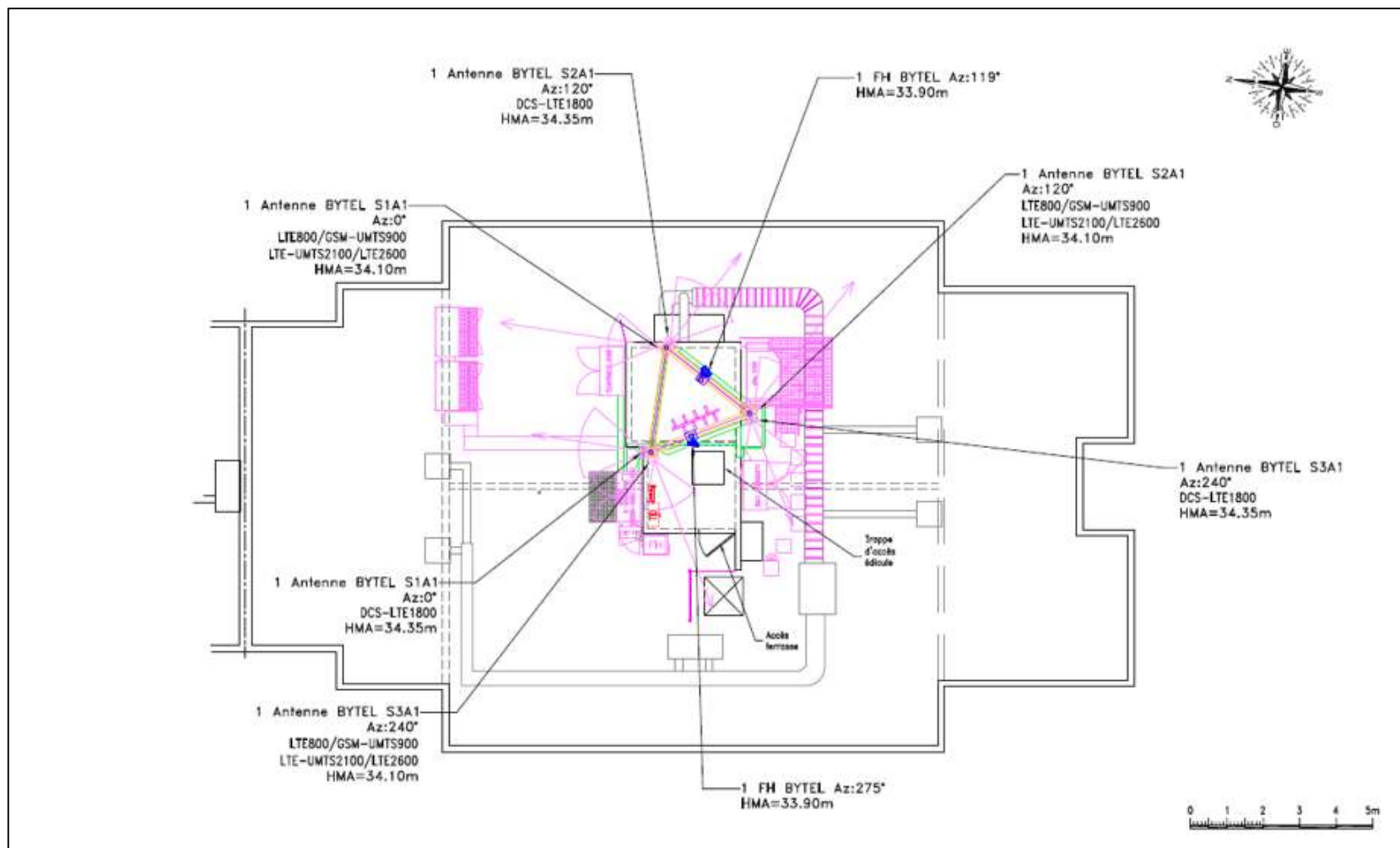
PLAN DE MASSE ETAT PROJETE
