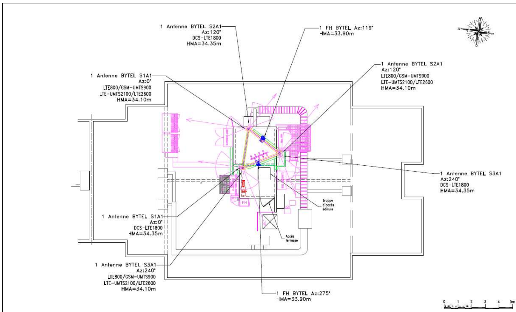
PLAN DE MASSE ETAT EXISTANT
