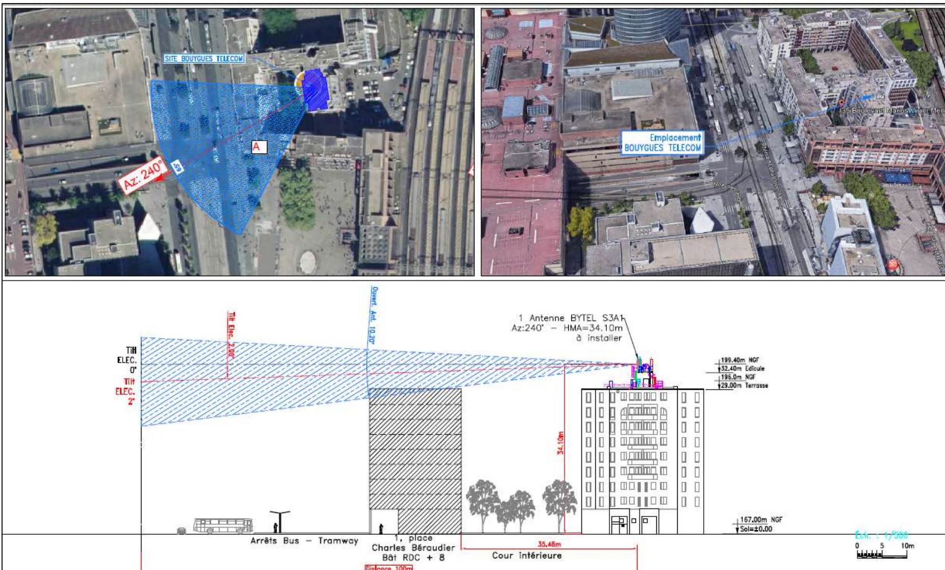
COUPE SUR L'AZIMUT 240°
