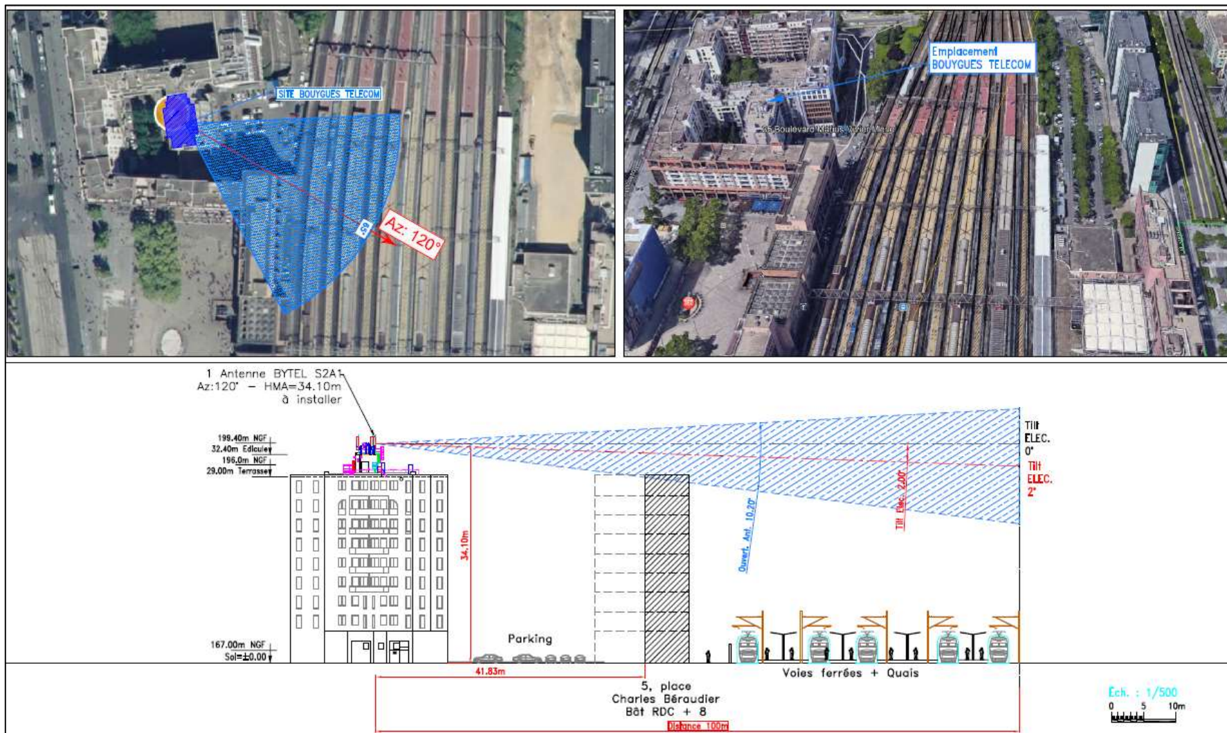
COUPE SUR L'AZIMUT 120°
