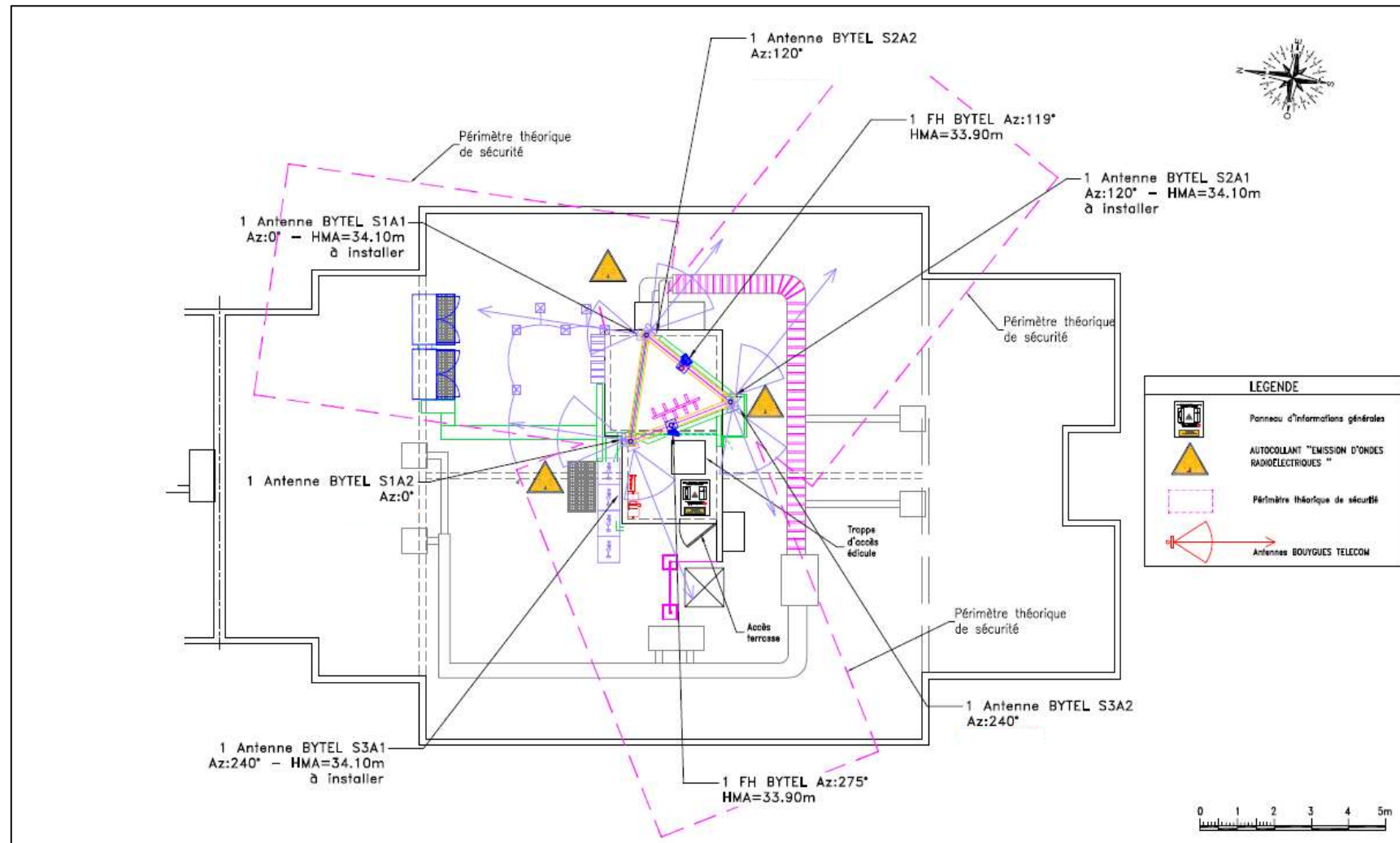
PERIMETRE DE SECURITE AUTOUR DES ANTENNES
